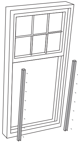
geen aanpassingen aan kozijn enkel vastschroeven van VR Strips in spinning
